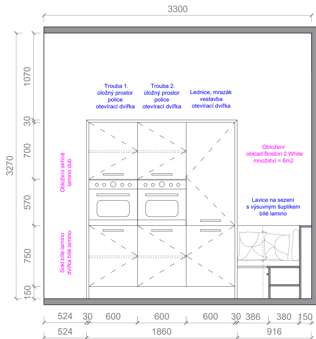
Pohled B - Boční stěna se spotřebiči
