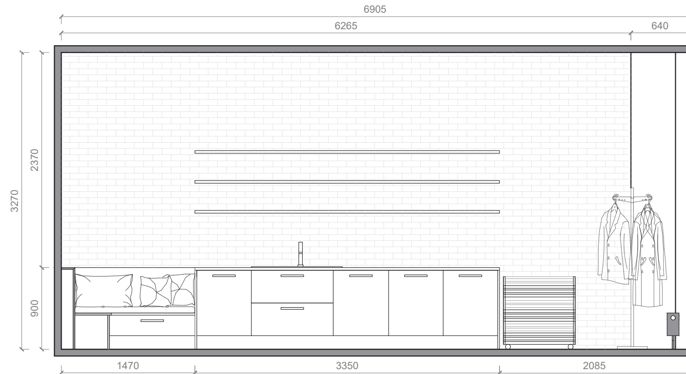
POHLED C - KUCHYNĚ - OSTRŮVEK, PŘEDNÍ ČÁST
