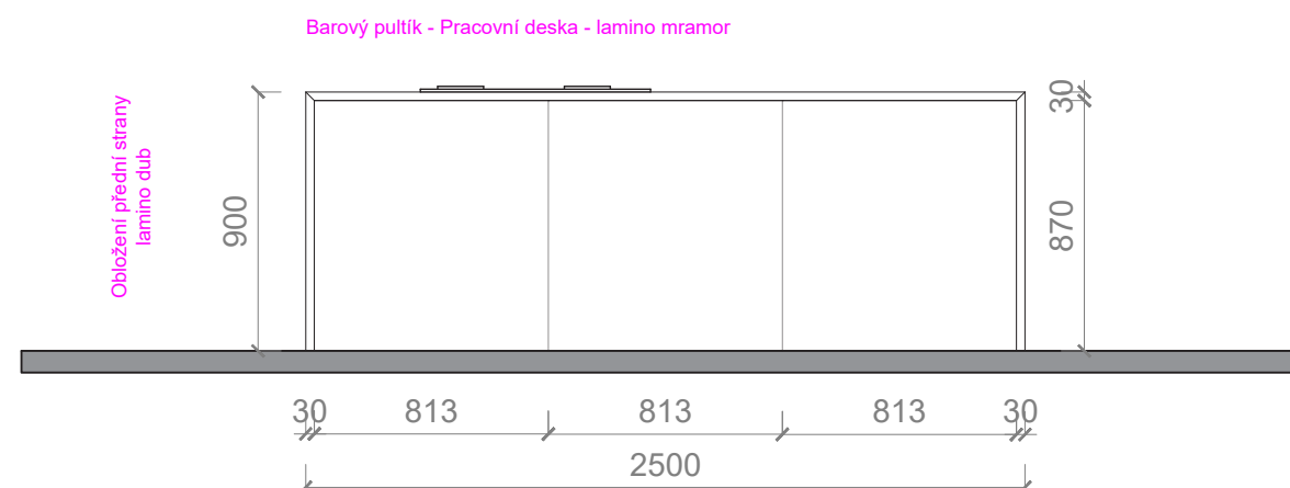
Pohled D - Ostrůvek, zadní část
