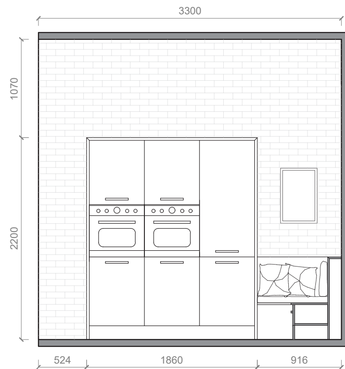
POHLED E - KUCHYNĚ - PŘEDNÍ STĚNA A OSTRŮVEK
