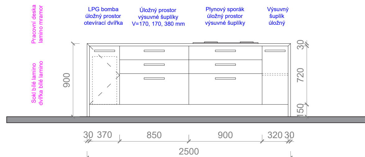
Pohled D - Ostrůvek, zadní část
