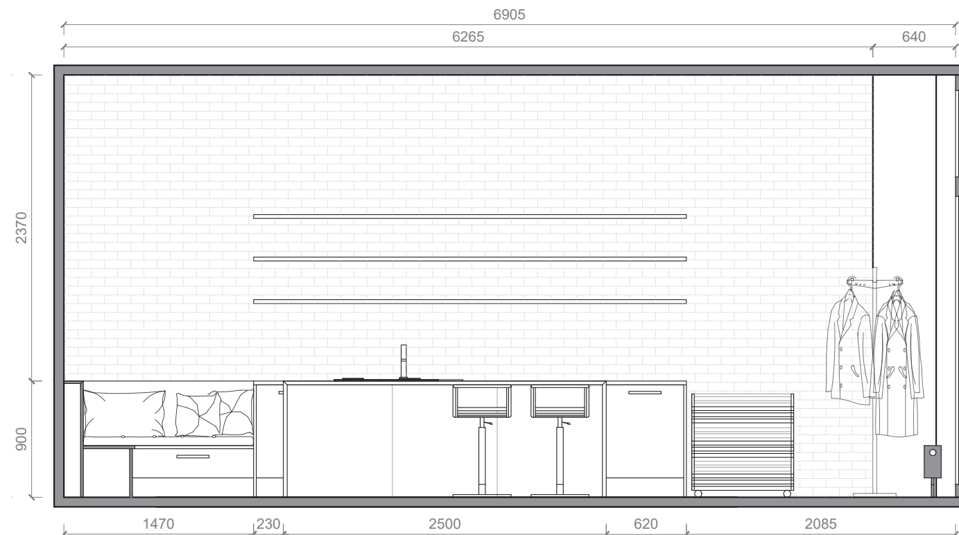
POHLED E - KUCHYNĚ - PŘEDNÍ STĚNA A OSTRŮVEK
