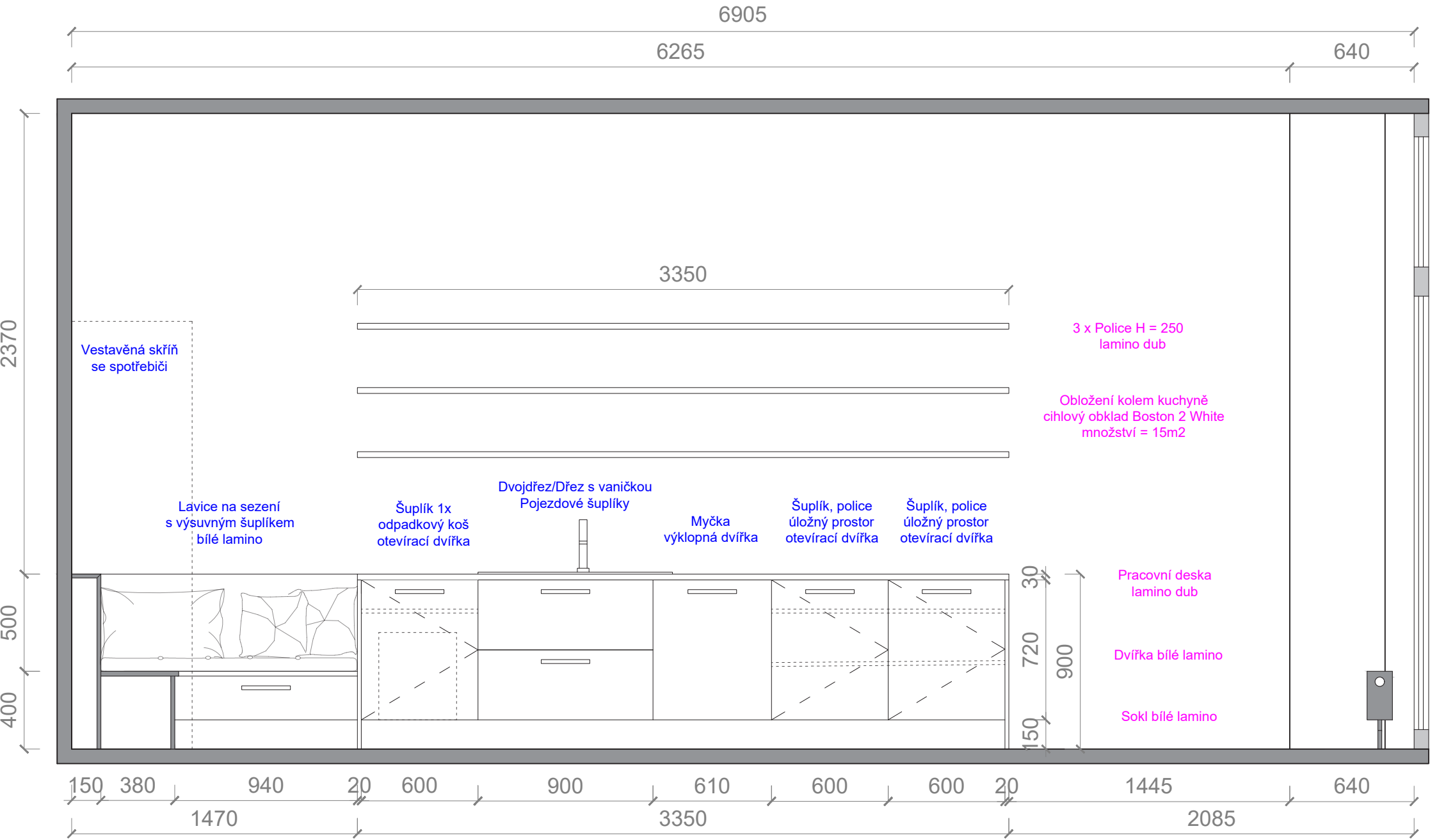
Pohled A - Kuchyně, přední stěna s policemi
